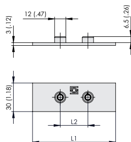
2 Schweißmuttern (B)
