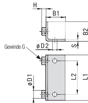
STAUFF Größe 1A bis 6 (7M / 8M)
