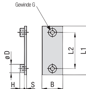
STAUFF Größe 1A bis 8 (7M / 8M)
