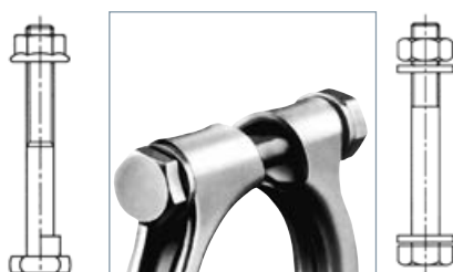
Version M10 und M12 mit Sechskantschraube.
